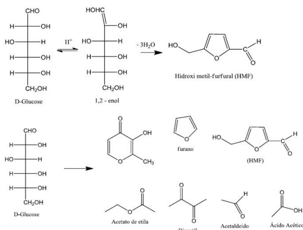
Figura 1. Esquema das reações que acontecem no processo de caramelização.
