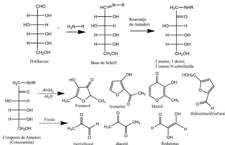
Figura 2. Esquema das reações que acontecem no processo conhecido como reações de Maillard .
